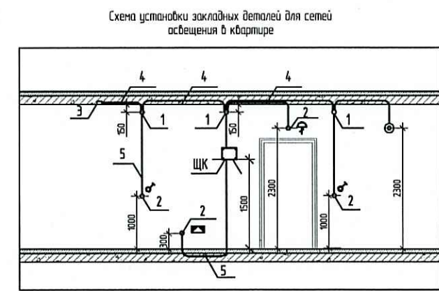
1 - Коробка ответвительная 2 - Коробка установочная 3 - Коробка установочная потолочная с клеммной колодкой для светильника 4 - Труба ПНД № 25 в монолитном перекрытии выходящая этажа для сетей освещения 5 - Труба ПНД № 20 в монолитном перекрытии бокового этажа для сетей уравнивания потенциала
