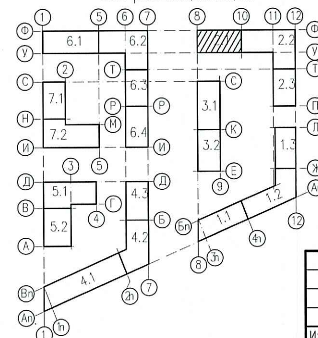
Схемарасположения
