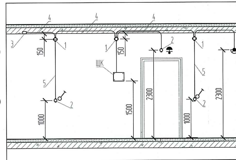
Схема установки накладных деталей для сетей освещения в квартирах
