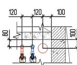
Прибязка стоек ВК к стенам
