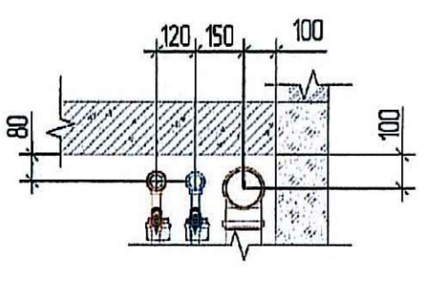
Привязка стояков ВК к стенам
