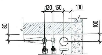
Привязка стояков ВК к стенам
