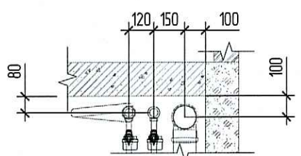
Прибытка стояков ВК к стенам
