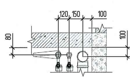
Приблизка стояков ВК к стенам
