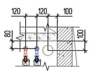
Приязка стояков ВК к стенам
