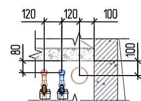
Привязка стояков ВК к стенам
