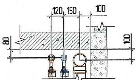
Приязка стояков ВК к стенам
