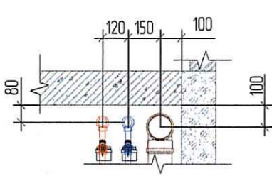
Приблизка стояков ВК к стенам
